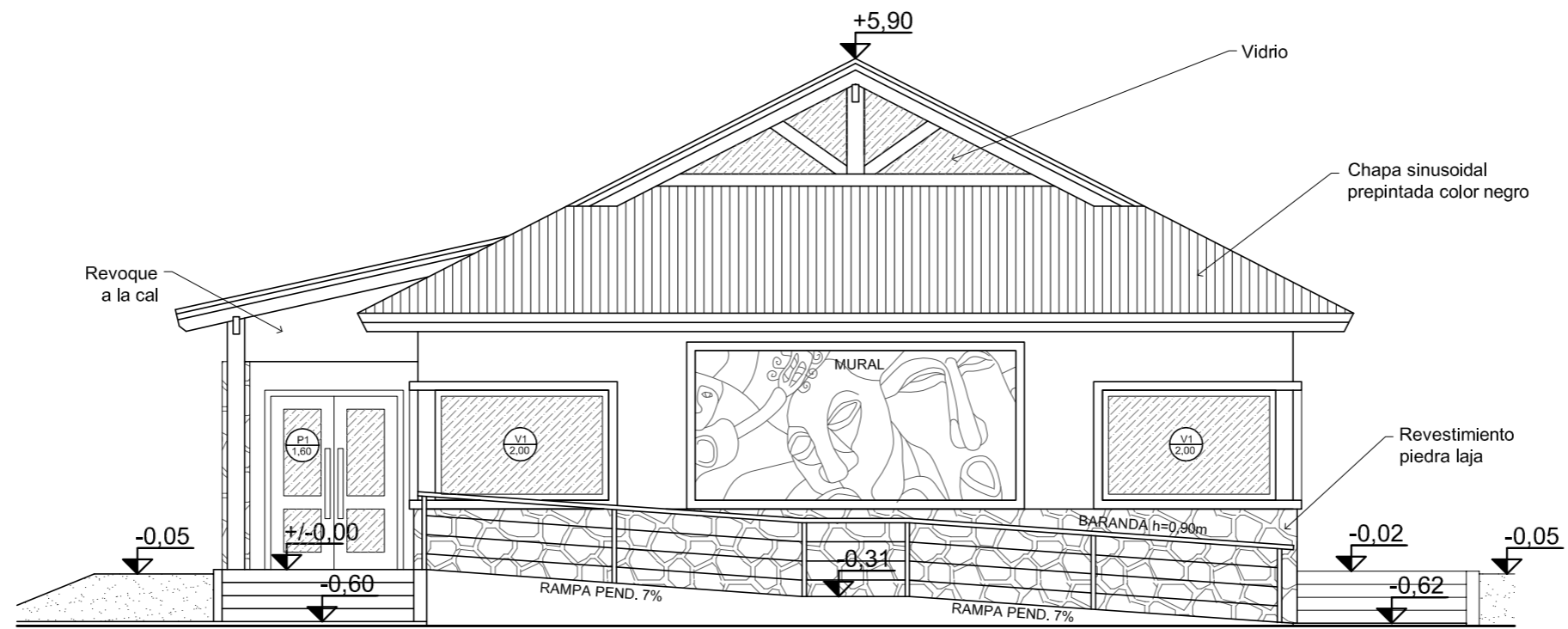
VISTA NOR-OESTE Esc. 1:75
