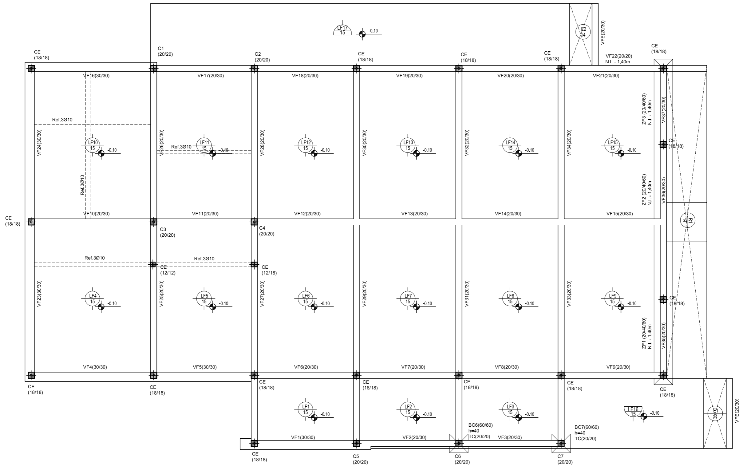
ESTRUCTURA PLATEA -0.10m
