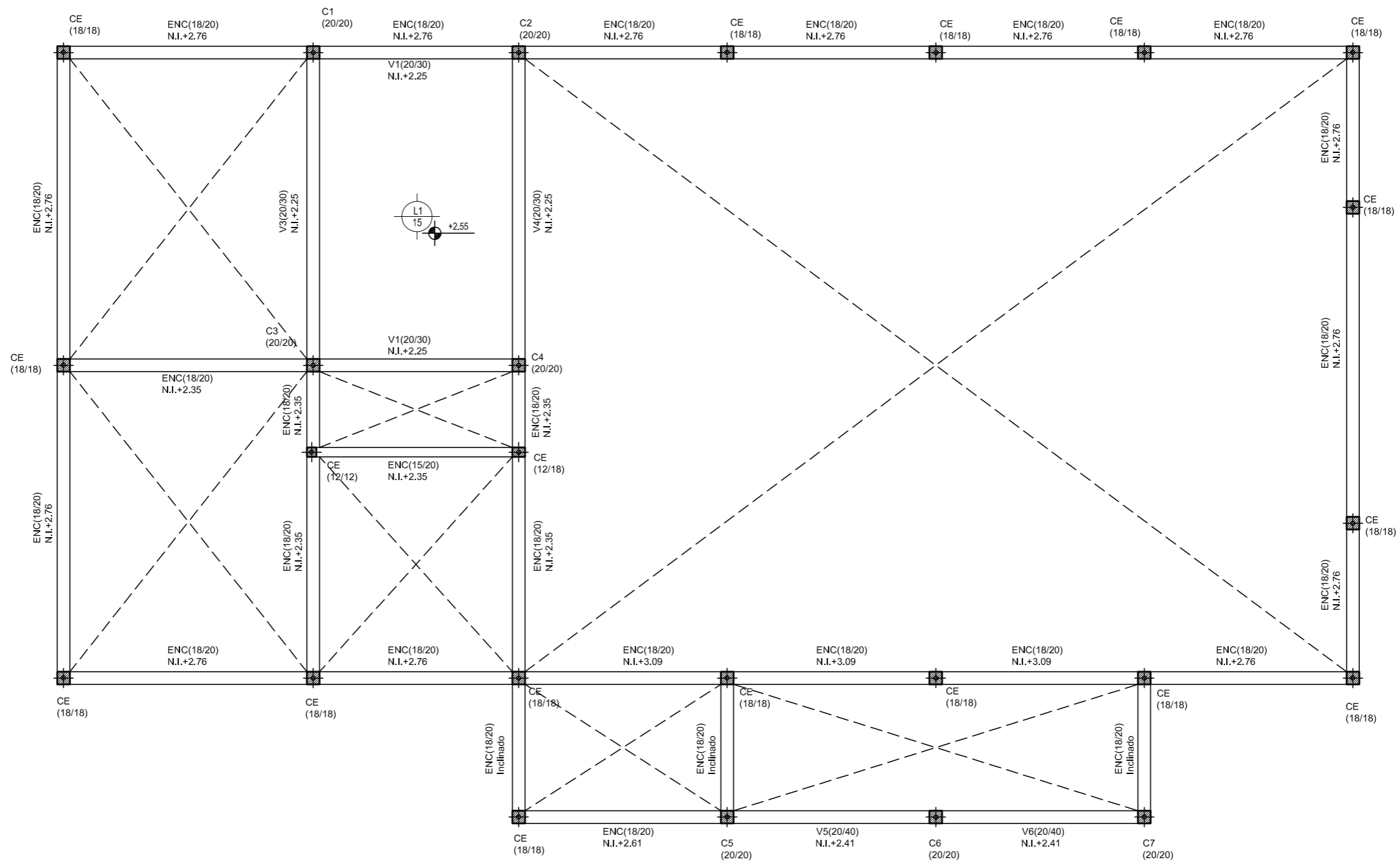
ESTRUCTURA S/PLANTA BAJA
