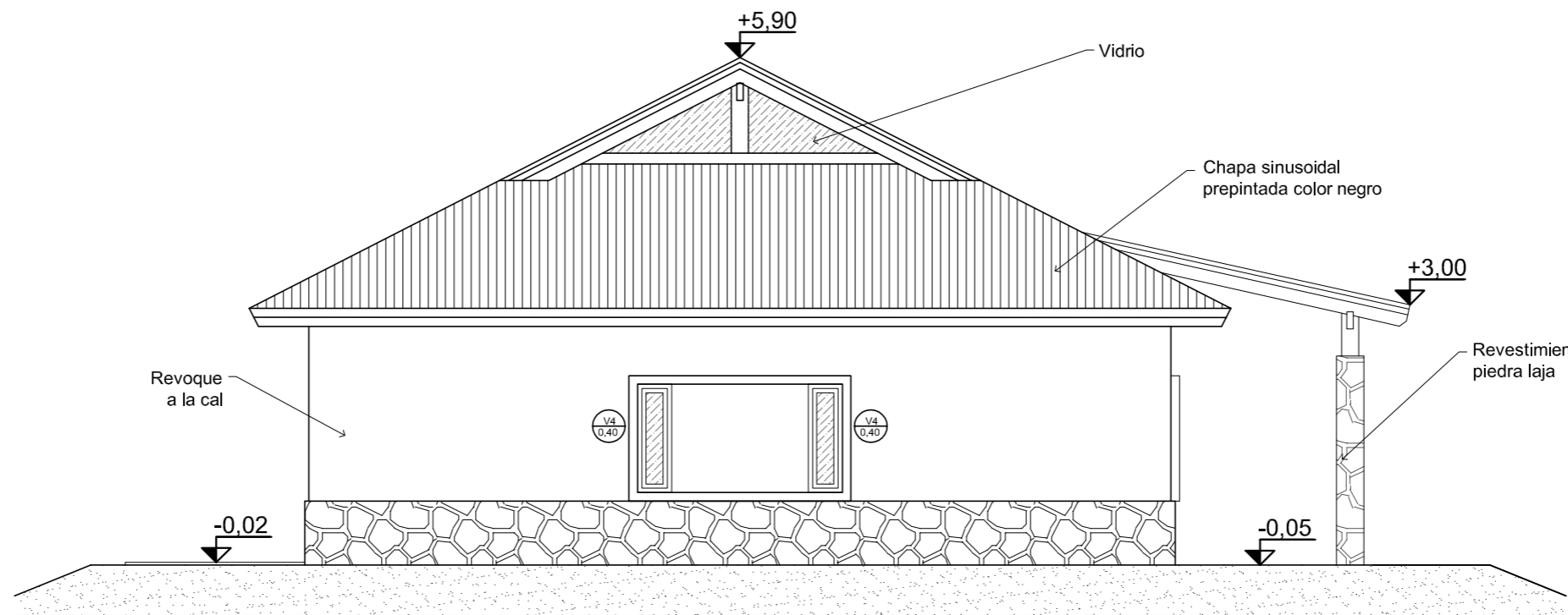
VISTA SUR-ESTE Esc. 1:75
