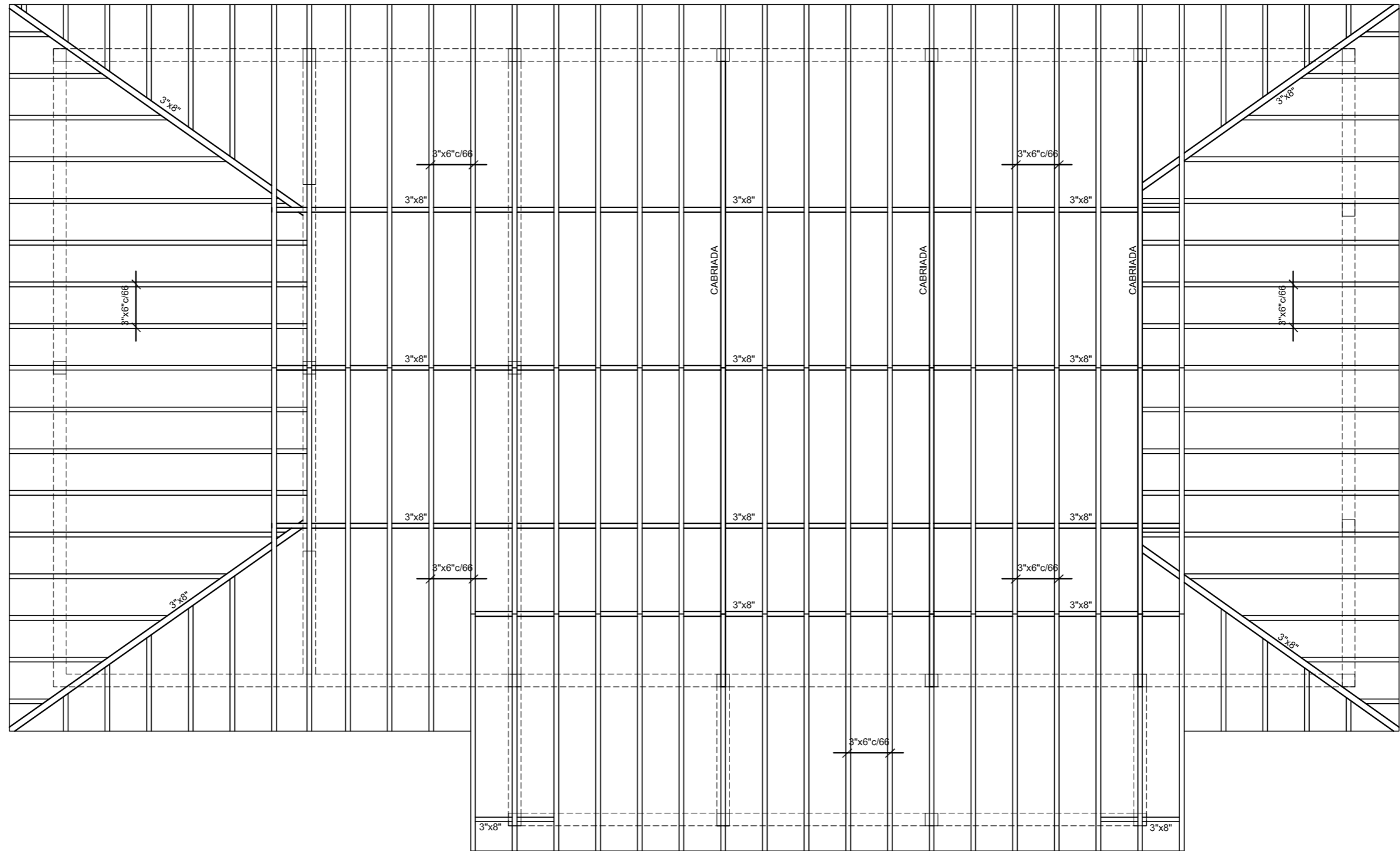
ESTRUCTURA DE TECHOS
