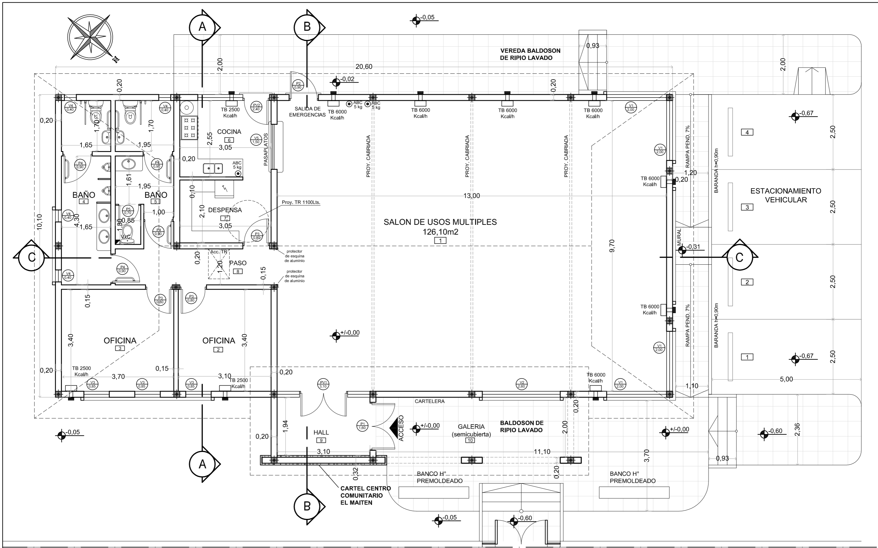
PLANTA BAJA Esc. 1:75
