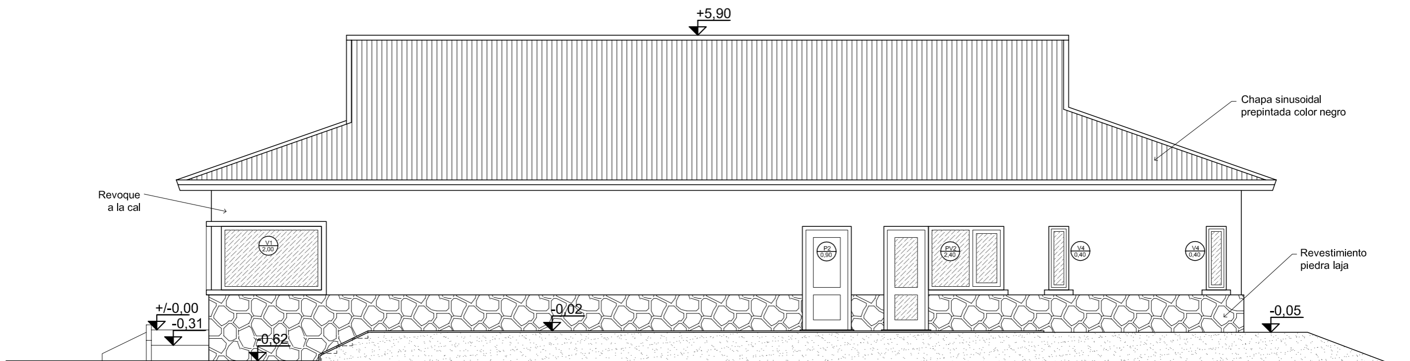
VISTA SUR-OESTE Esc. 1:75
