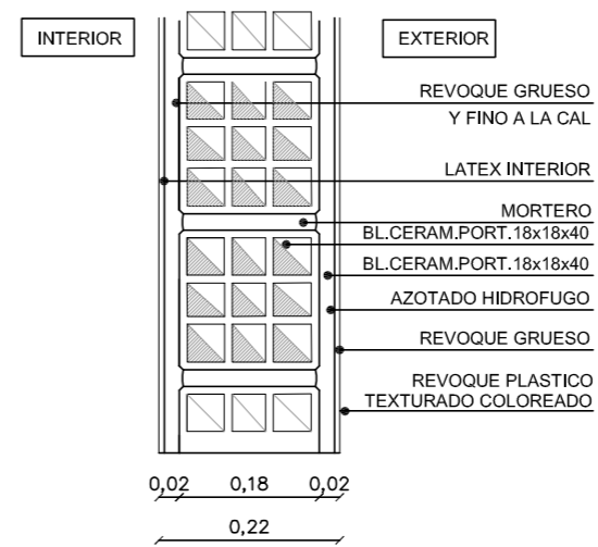
DETALLE MAMPOSTERIA ESC. 1:10
