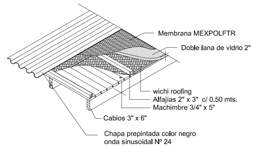
DETALLE DE CUBIERTA
