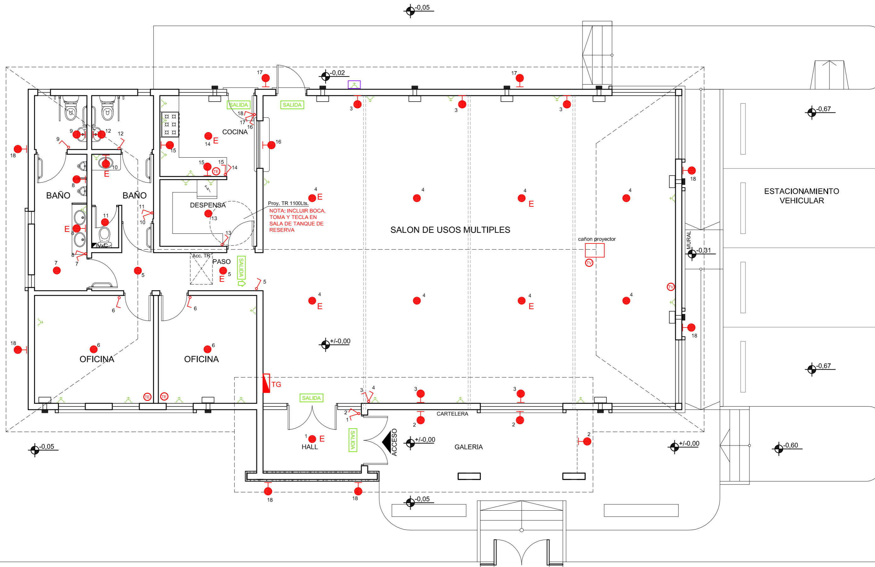
PLANTA BAJA Esc. 1:75 ESQUEMA DE DISTRIBUCION DE INSTALACIONES ELECTRICAS
