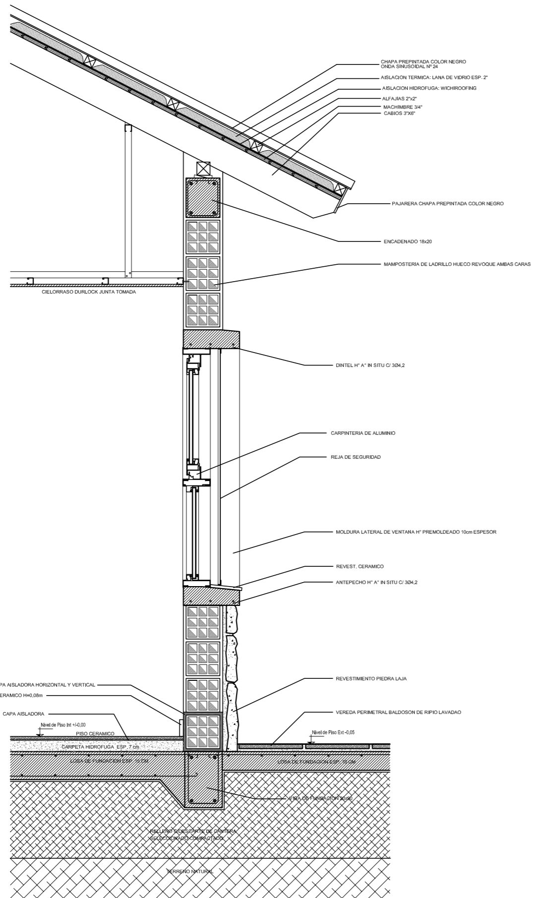
CORTE CONSTRUCTIVO ESC. 1:20
