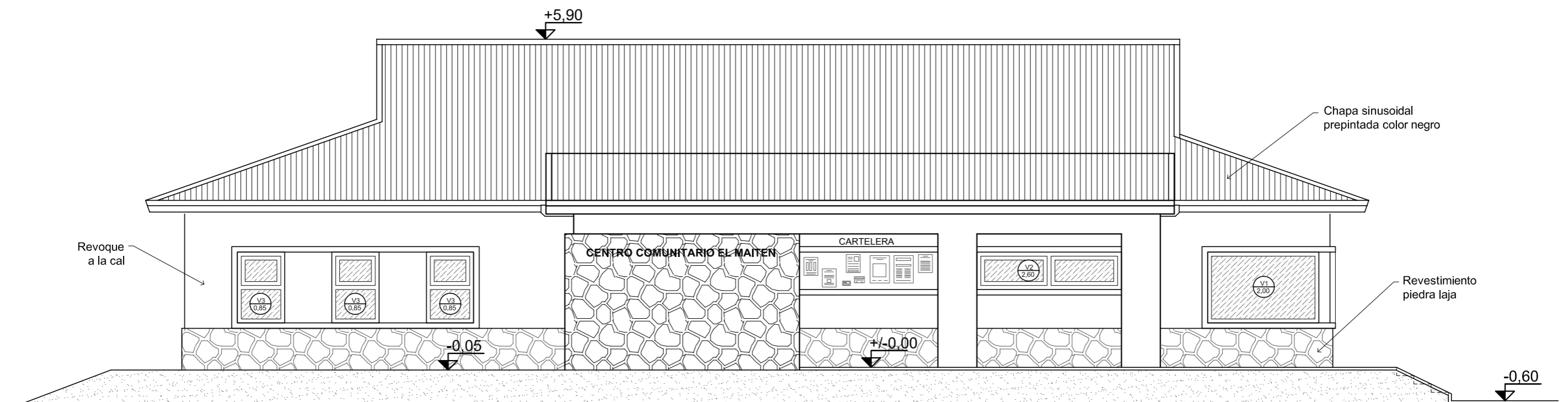
VISTA NORT-ESTE Esc. 1:75
