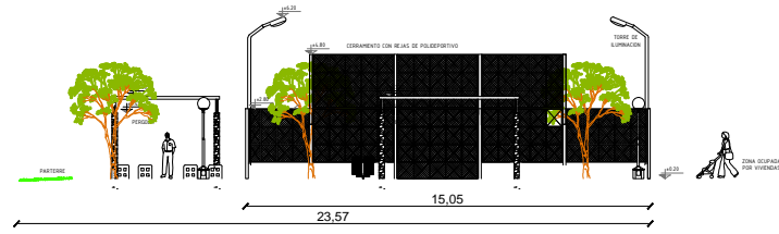
VISTA DE FRENTE
