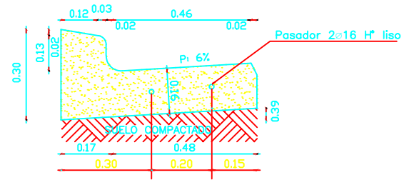
Ubicación de pasadores en junta de expansión
