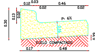
Detalle cordón cuneta
