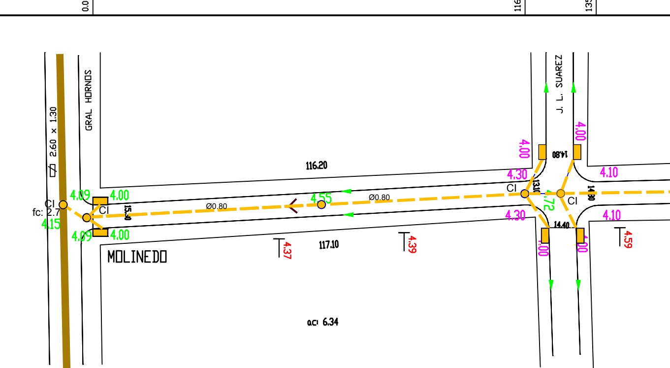
MOLINEDO ENTRE GRAL HORNOS y SAN JOSE
