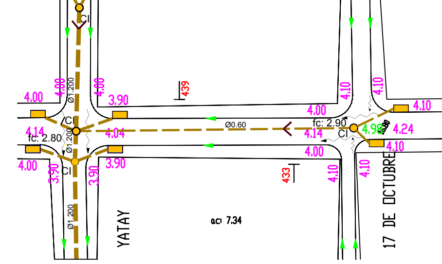
MAGALLANES ENTRE YATAY y 17 de OCTUBRE
