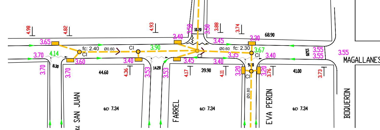
MAGALLANES ENTRE SAN JUAN y EVA PERON
