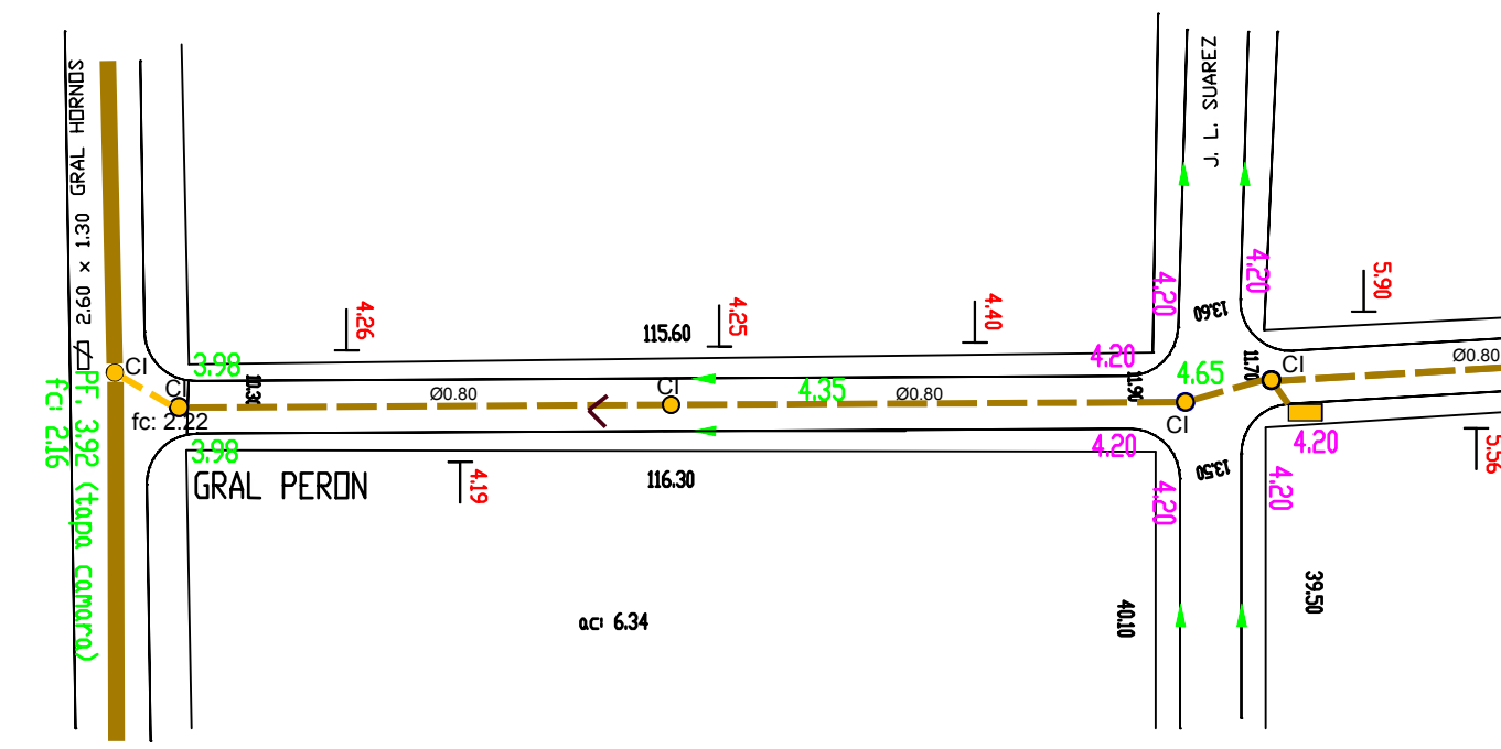
GRAL PERON ENTRE GRAL HORNOS y SAN JOSE
