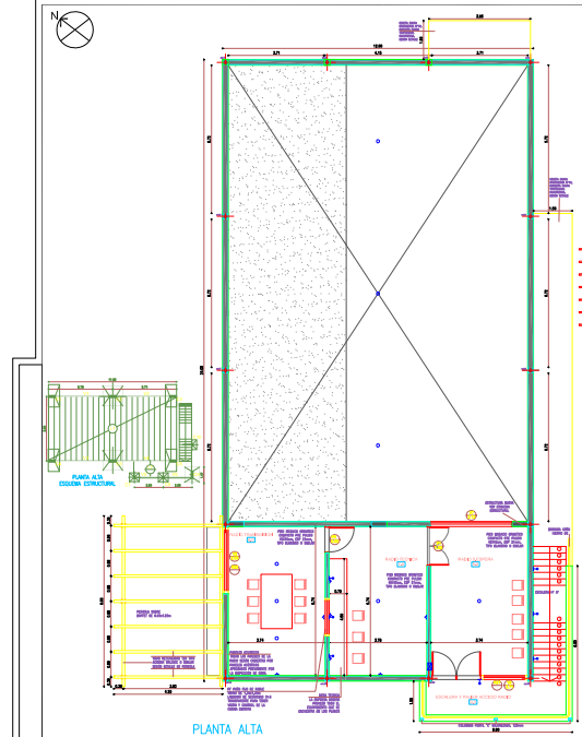
PLANTA ALTA
