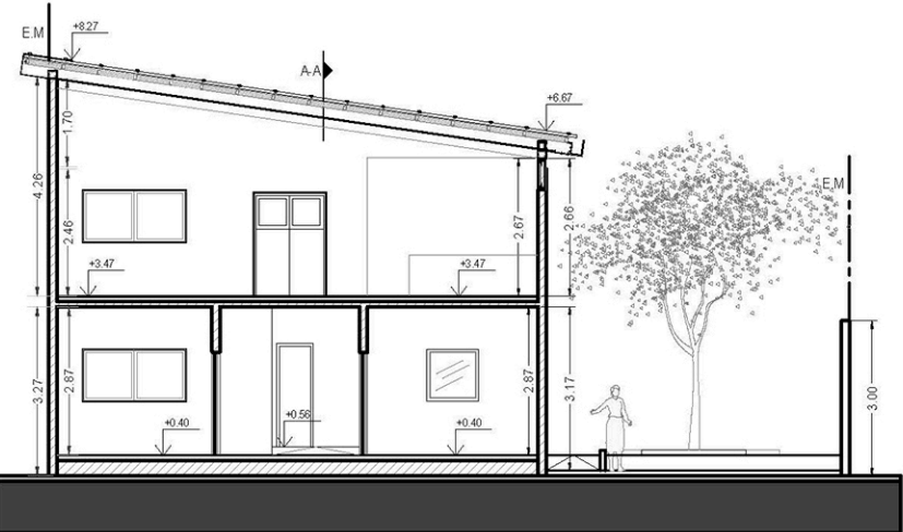
CORTE B-B
