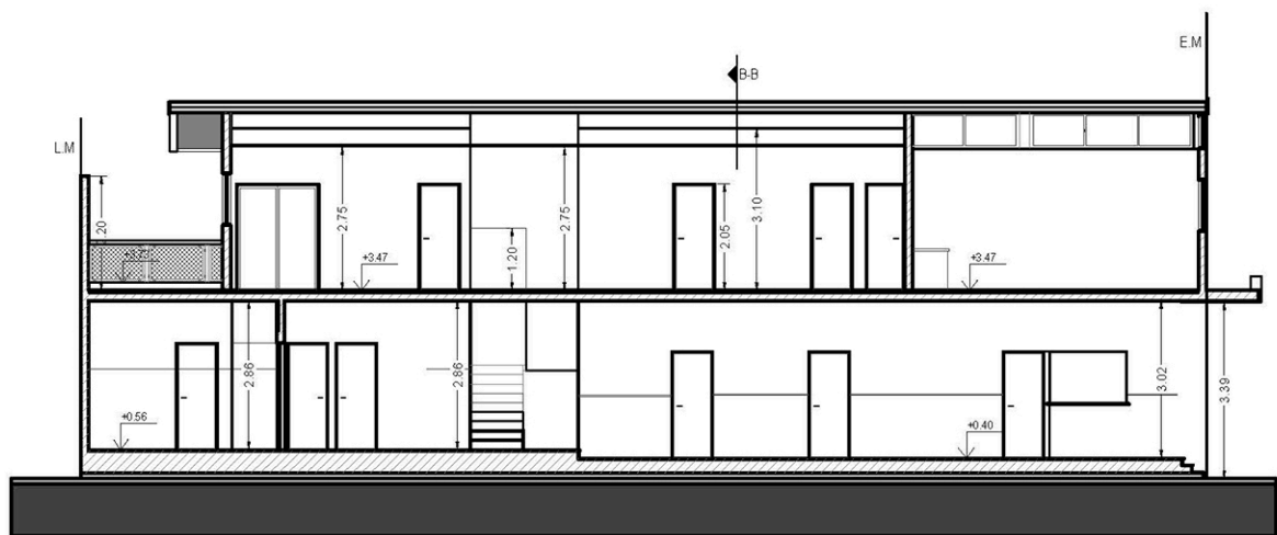
CORTE A-A
